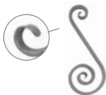
Ref. \updownarrow \leftrightarrow \blacksquare 05163 300 x 150 16x8 05164 400 x 150 16x8 05165 400 x 200 16x8 05166 500 x 200 16x8 05167 600 x 250 16x8 05168 750 x 250 16x8
