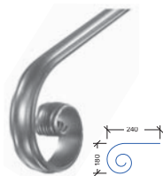
Rfe. medidas en m/m Ref. ↓ ↑ ↕ ↔ ↘ ↙ 03149 180 x 400 50x14 03149.03 180 x 400 40x12
